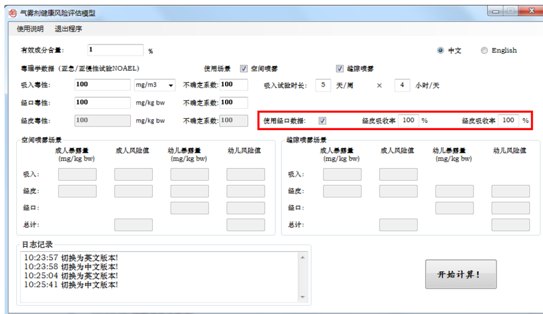
图 6. 经皮毒性
