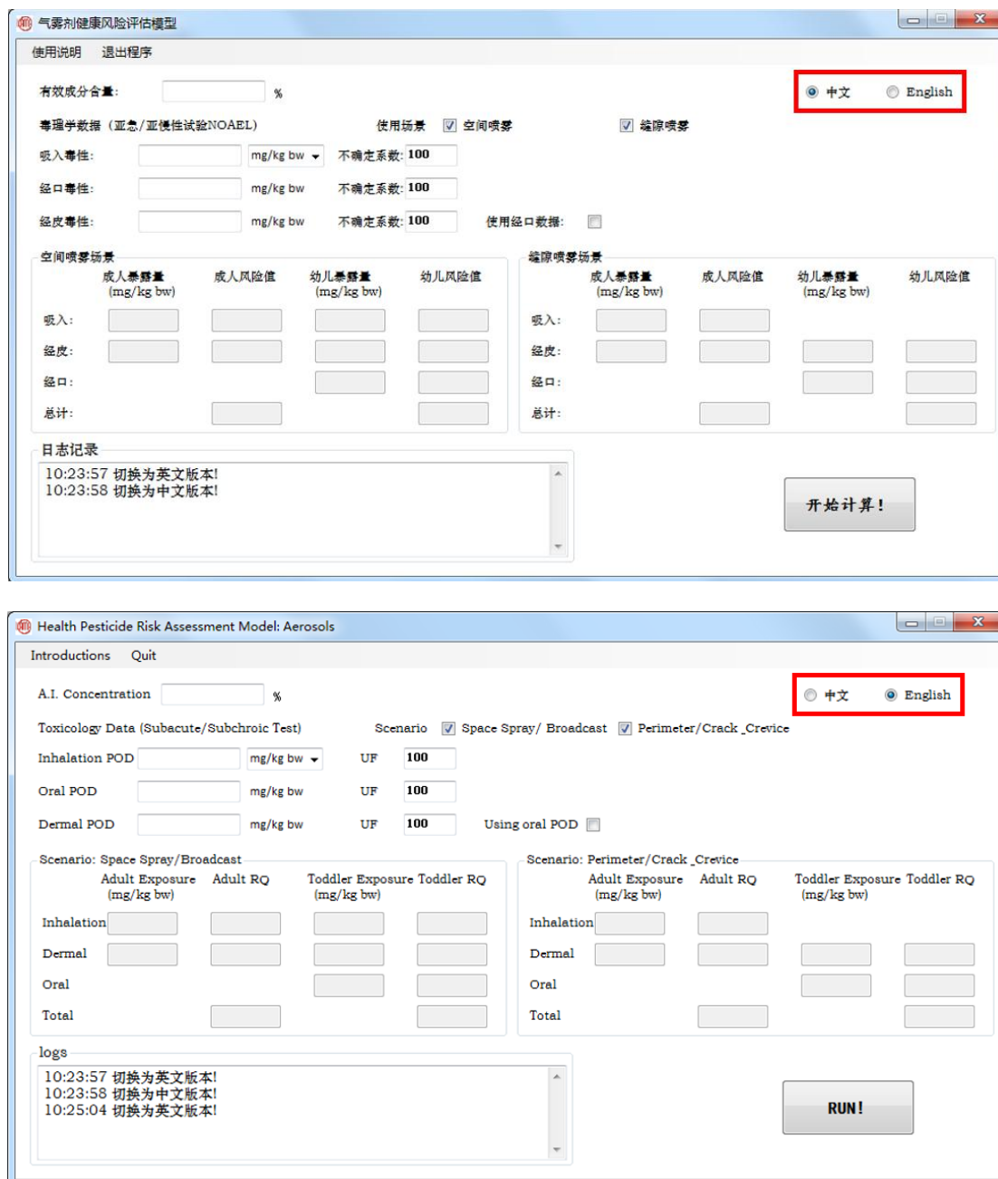
图 1. 软件主界面
