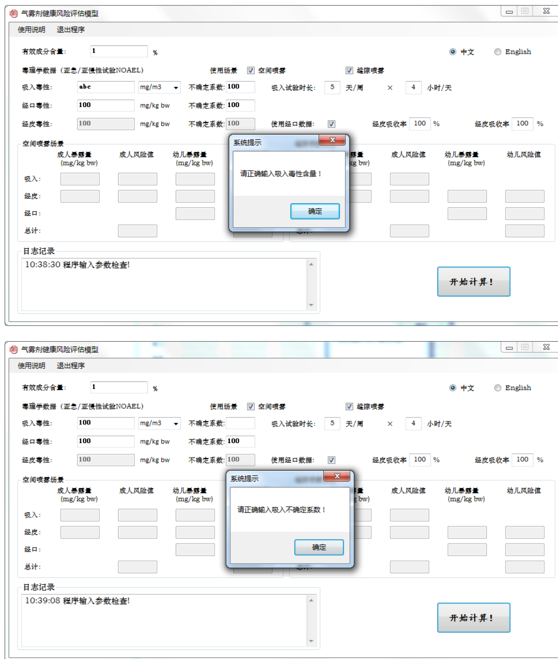
图 7. 开始计算
