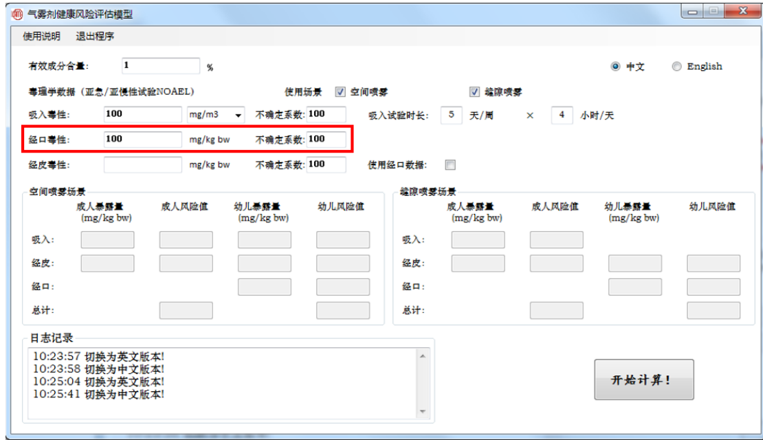
图 5. 经口毒性
